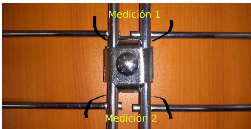
Foto N°1: Muestra ensayada
