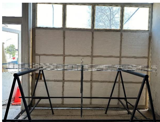
Foto N°2: Montaje utilizado
