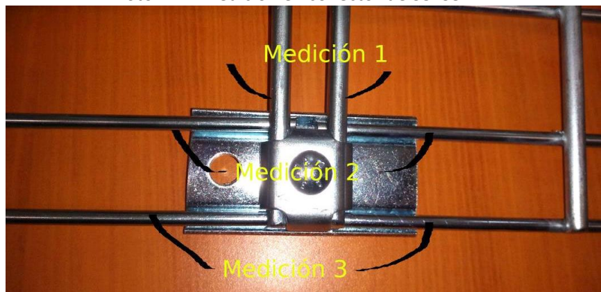
Foto Nº3: Medición en conector de 44x80 mm
